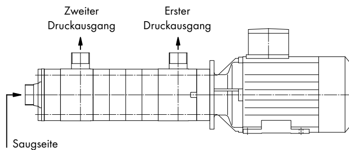
Abb.: Pumpe Typ ZHB 32-08
